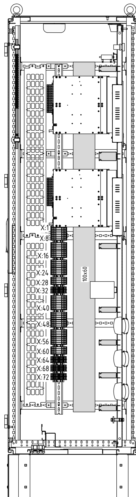
Г-Г
